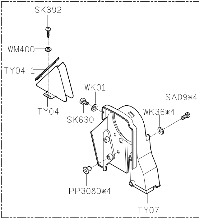
TY07-A 手輪護蓋
